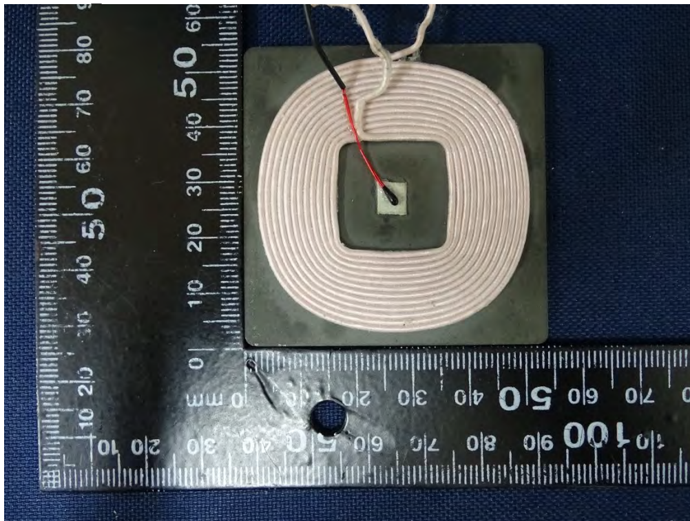
(46) EUT Photo WPT Antenna
