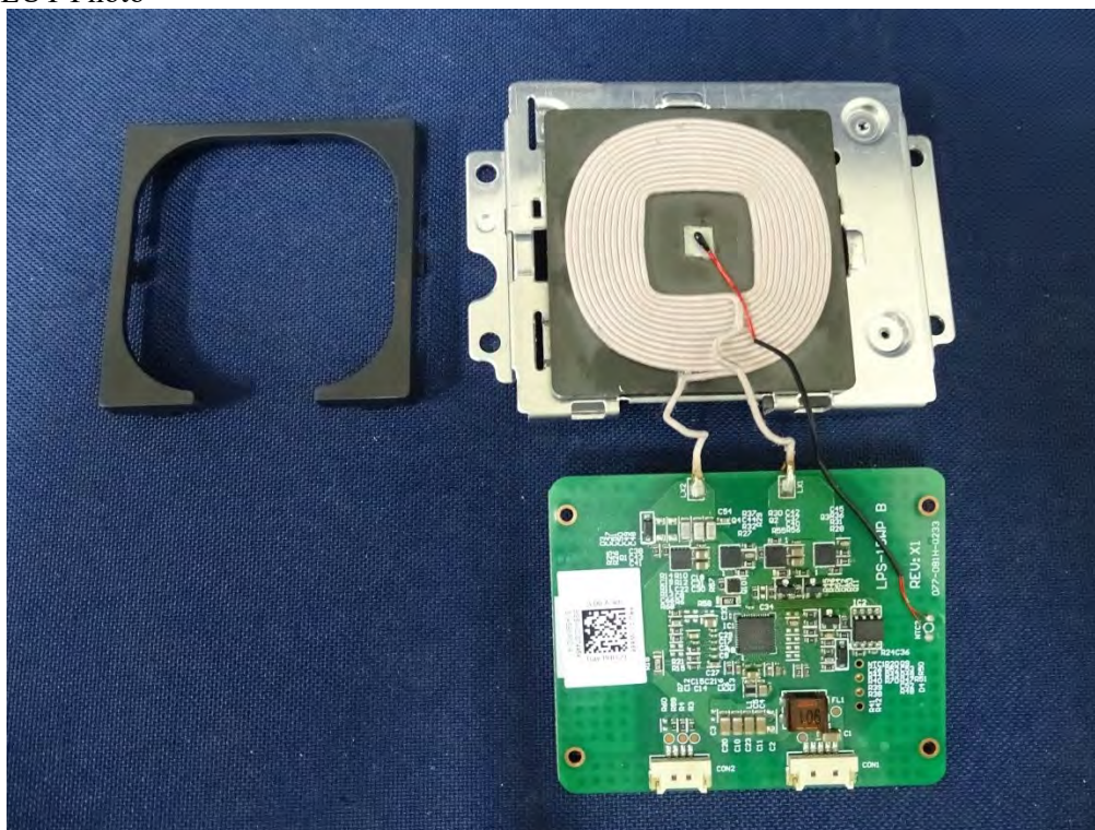
(41) EUT Photo
