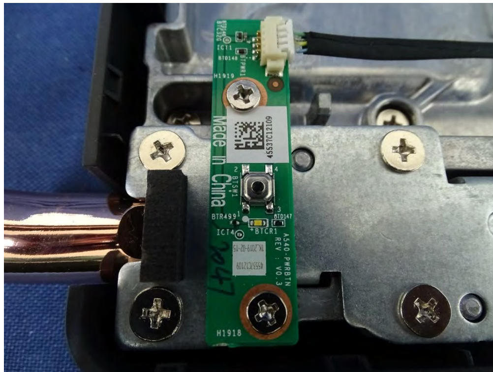
(36) EUT Photo
