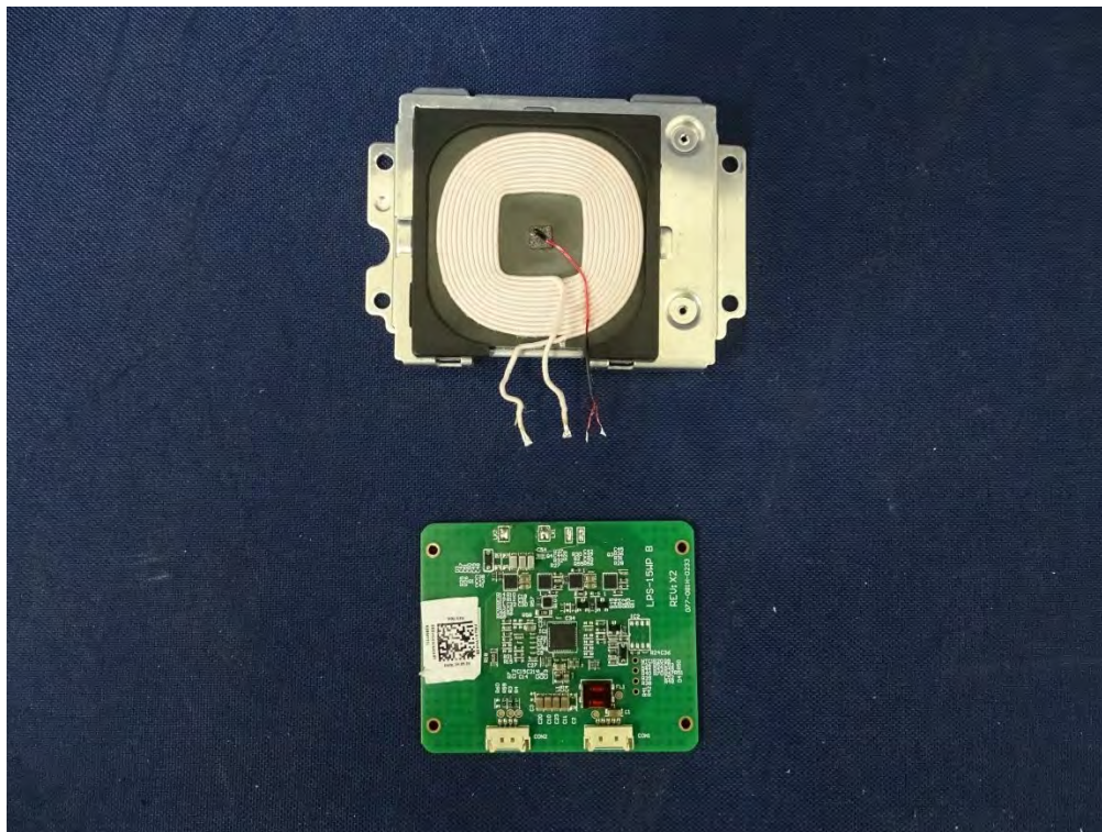
(44) EUT Photo
