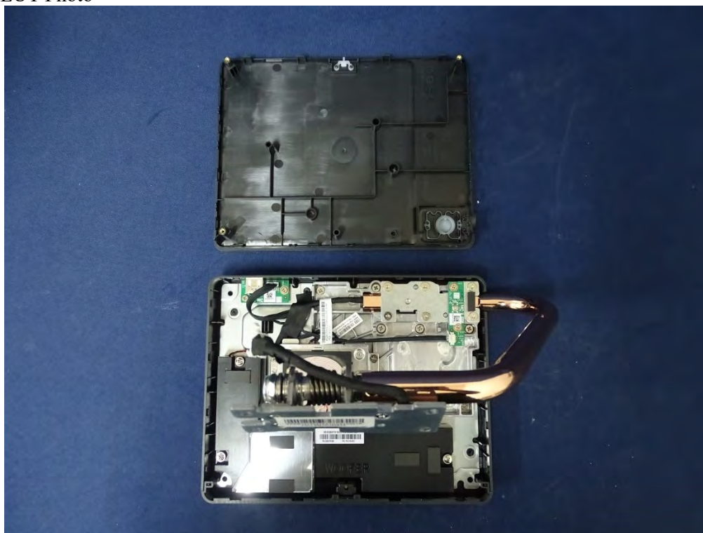
(33) EUT Photo
