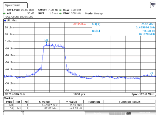
n20_2462MHz_Chain 0 45.03dB
