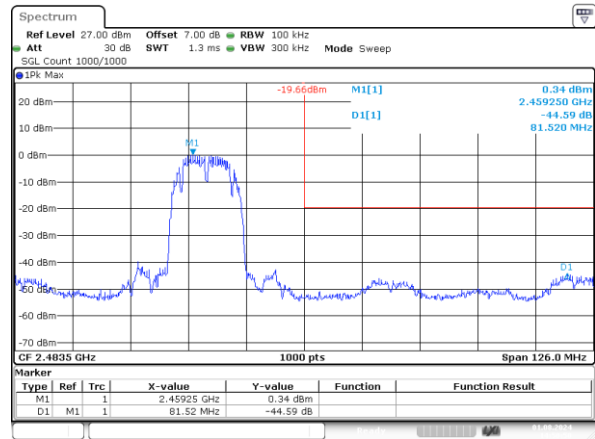
b_2462MHz_Chain 0 44.59dB
