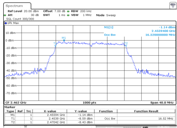
g_2462MHz_Chain 0 16.520MHz
