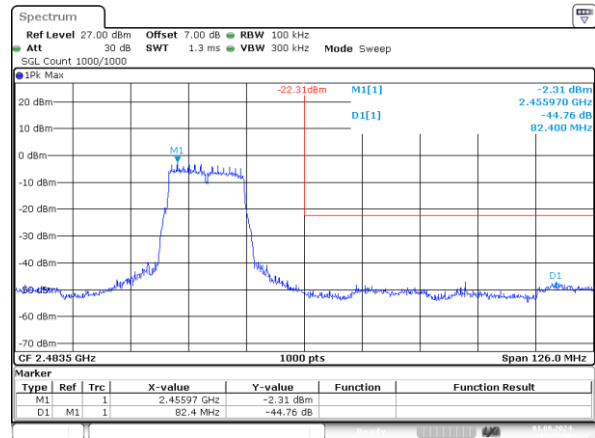
g_2462MHz_Chain 0 44.76dB
