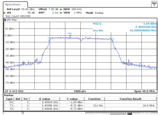
g_2412MHz_Chain 0 16.600MHz
