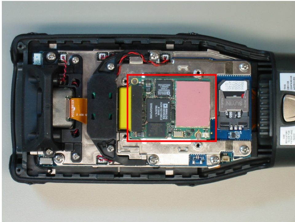
GSM Radio Module
