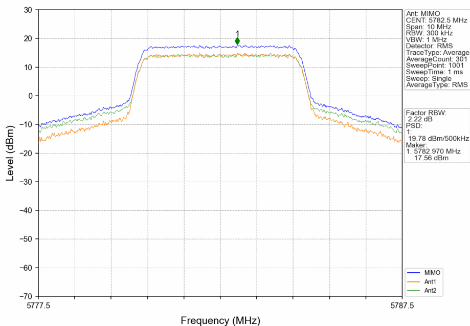
5M_MCH_5782.5MHz_MIMO_NTNV
