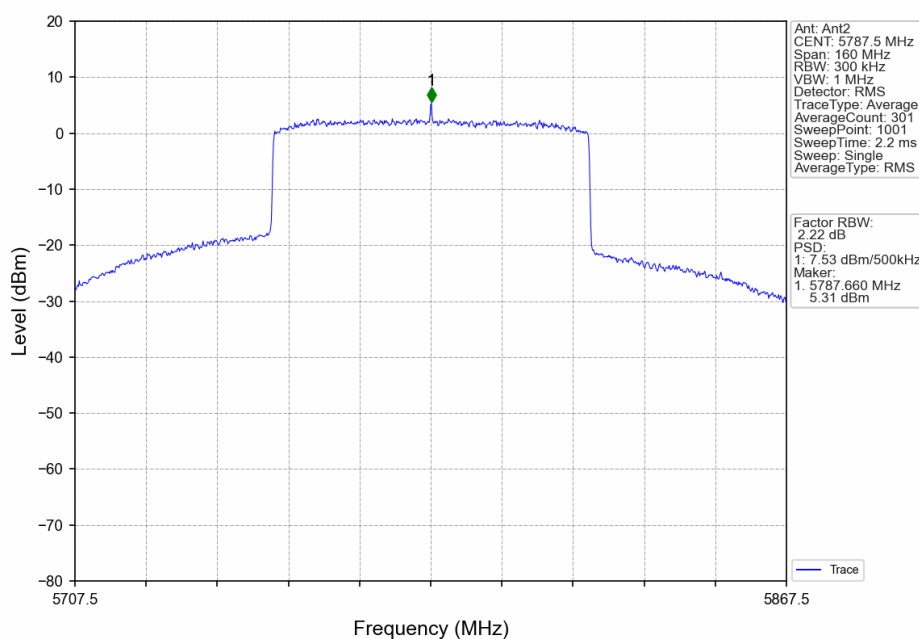
80M_MCH_5787.5MHz_Ant2_NTNV
