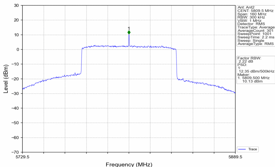
80M_HCH_5809.5MHz_MIMO_NTNV
