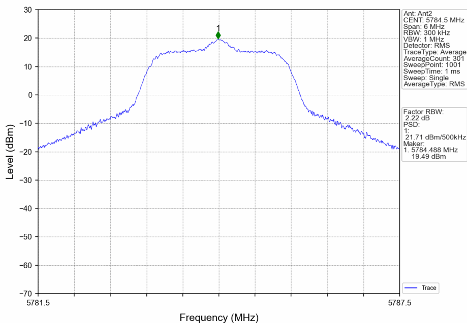
3M_MCH_5784.5MHz_Ant2_NTNV
