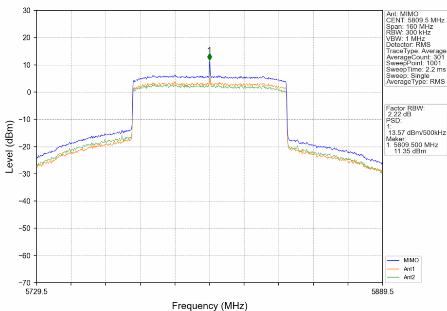
80M_HCH_5809.5MHz_MIMO_NTNV
