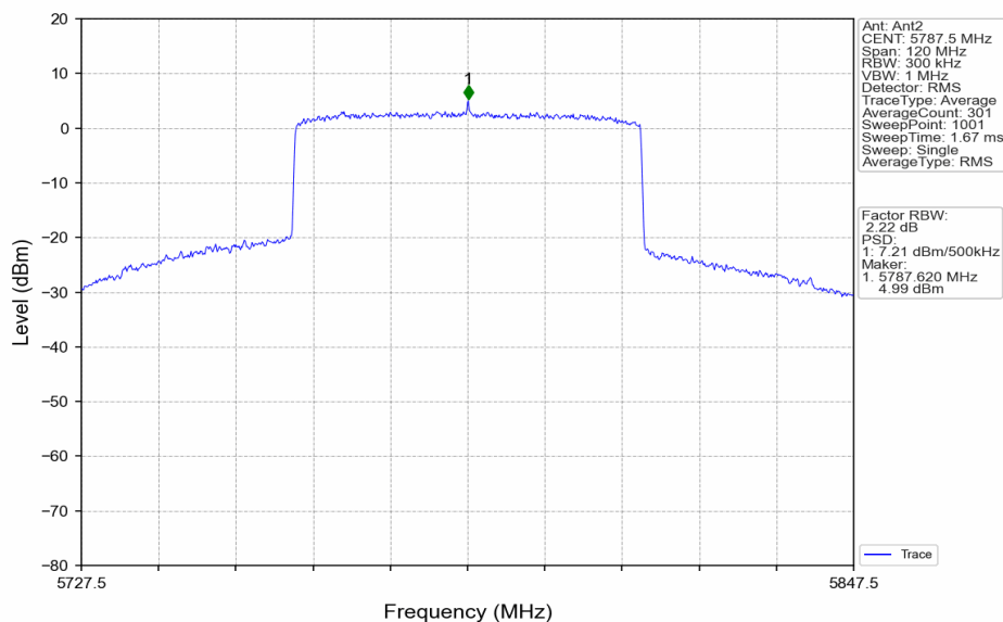
60M_MCH_5787.5MHz_MIMO_NTNV
