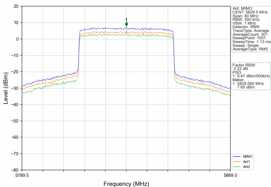
40M_HCH_5829.5MHz_MIMO_NTNV
