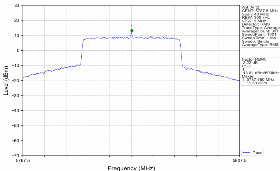
20M_MCH_5787.5MHz_MIMO_NTNV
