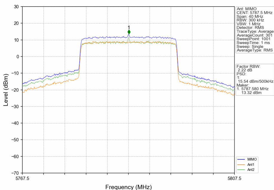
20M_MCH_5787.5MHz_MIMO_NTNV
