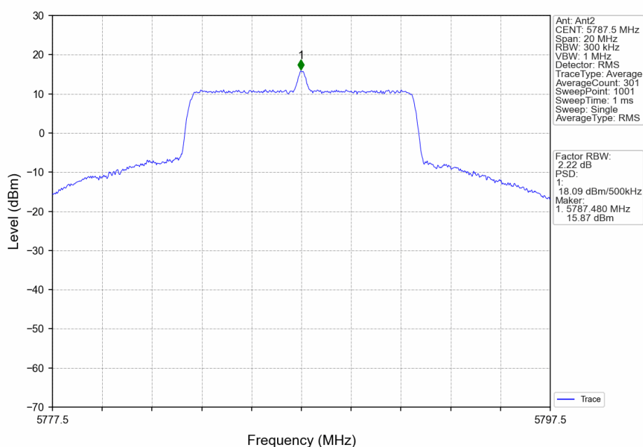
10M_MCH_5787.5MHz_Ant2_NTNV
