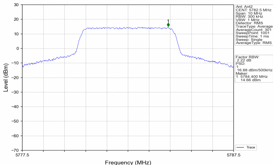
5M_MCH_5782.5MHz_MIMO_NTNV
