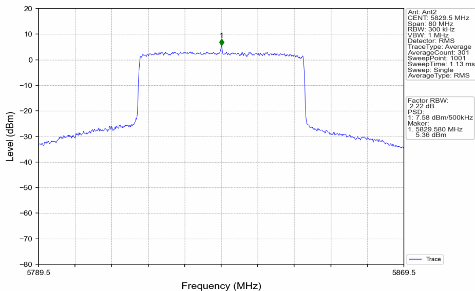
40M_HCH_5829.5MHz_MIMO_NTNV
