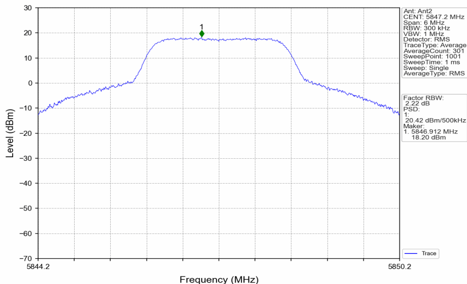
3M_HCH_5847.2MHz_MIMO_NTNV
