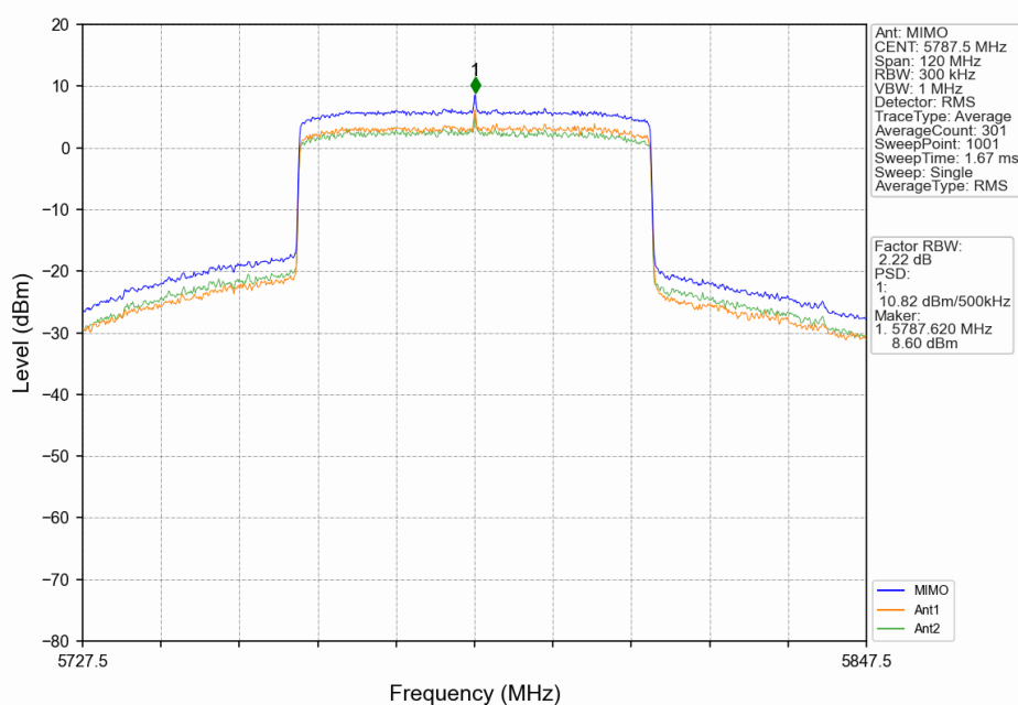
60M_MCH_5787.5MHz_MIMO_NTNV
