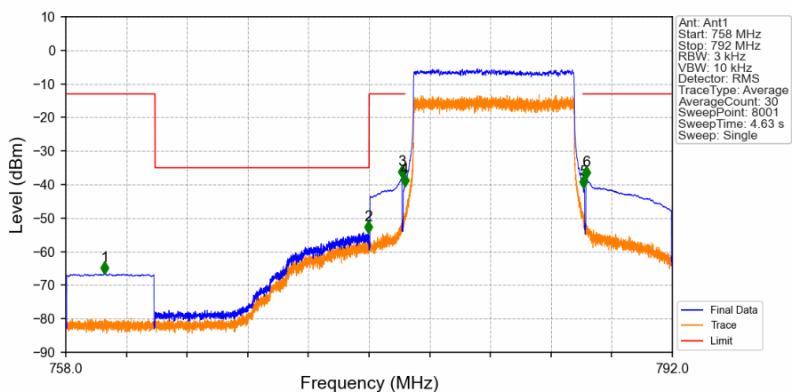
Band13 10MHz 16QAM LCH 782MHz RB 50 0 NTNV
