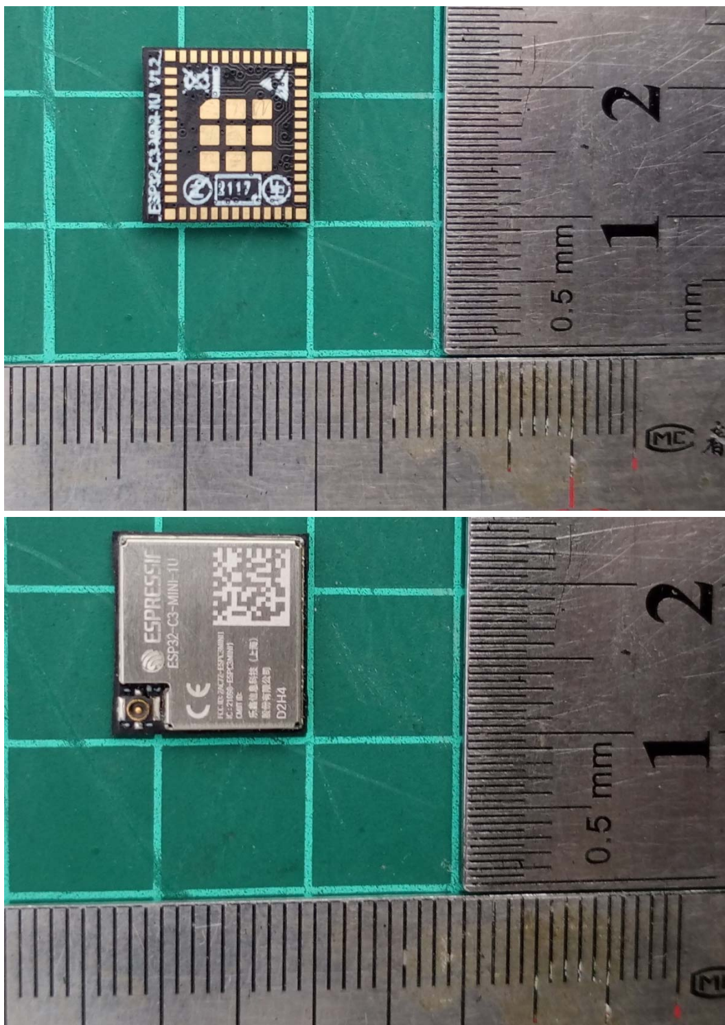
a: EUT
