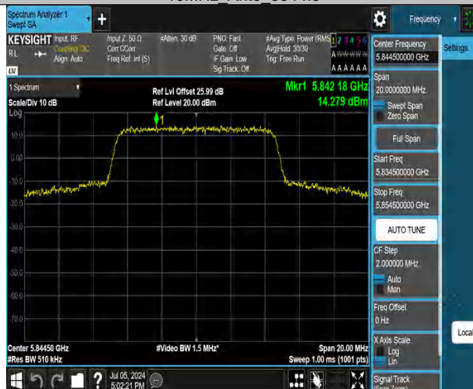
10MHz Ant6 5844.5
