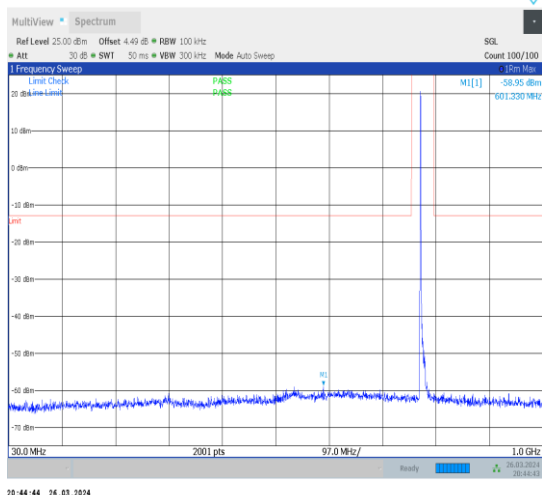
1-N13-15-10-H-1-DFT-PI2BPSK-Inner_1RB_Left-1 @1-30-1000-Ant1-601.33--58.95--13-PASS
