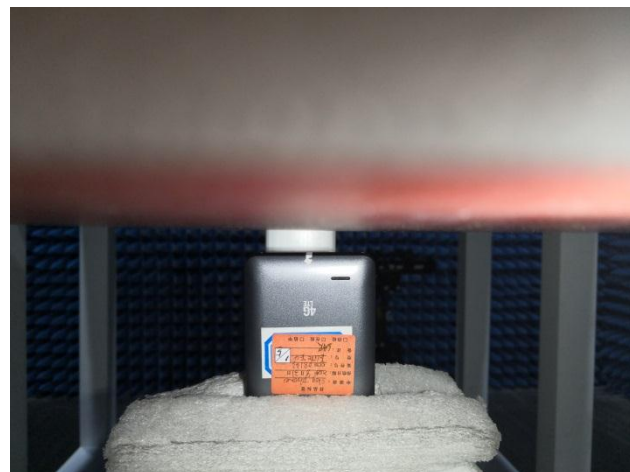
Bottom side(10mm)
