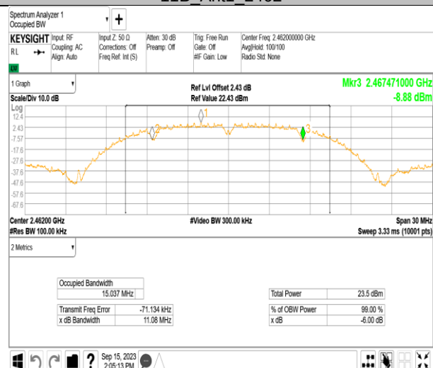
11B_Ant1_2462
