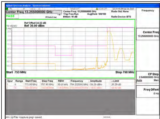
Band14 / 10MHz / Low CH / QPSK / 1 RB
