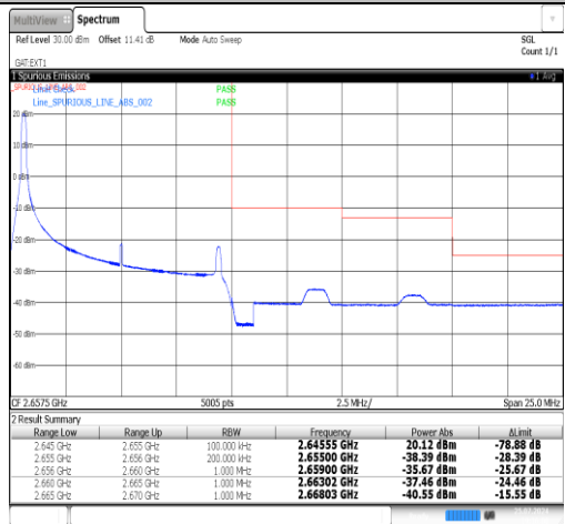
Band41(2535-2655)-10MHz-QPSK-41190-1RB#0-PASS
