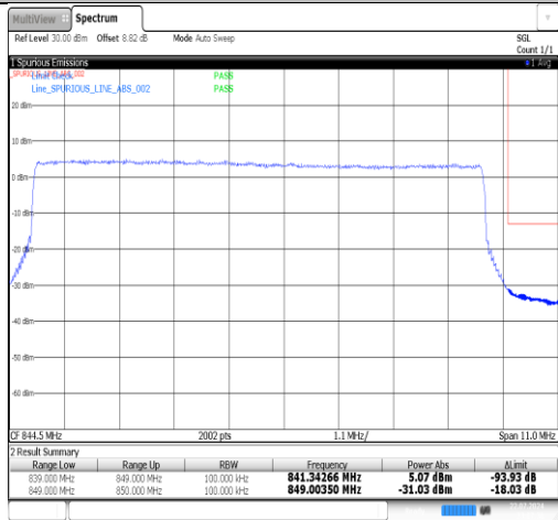
Band26(824-849)-10MHz-QPSK-26990-50RB#0-PASS
