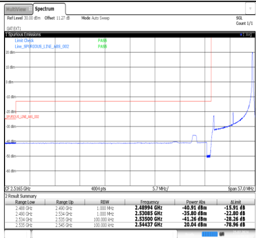
Band41(2535-2655)-10MHz-QPSK-40090-1RB#49-PASS
