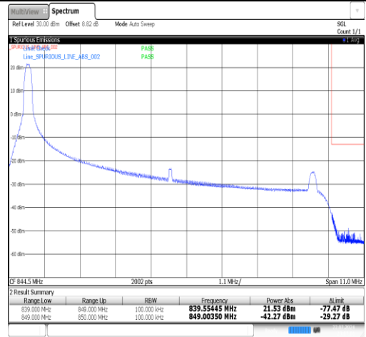
Band26(824-849)-10MHz-QPSK-26990-1RB#0-PASS
