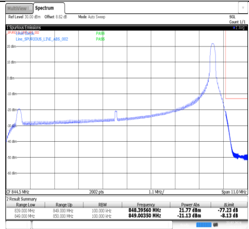
Band26(824-849)-10MHz-QPSK-26990-1RB#49-PASS
