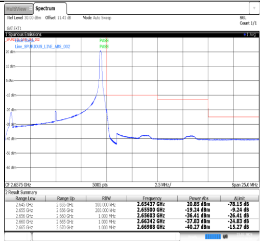
Band41(2535-2655)-10MHz-QPSK-41190-1RB#49-PASS
