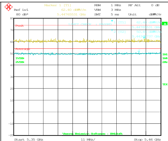
802.11n-HT20 5320M(5350-5460MHz)
