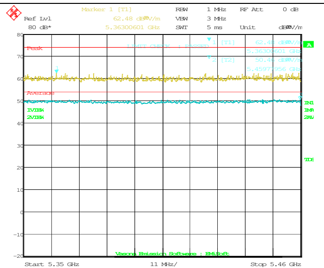
802.11ac 5530M(5350-5460MHz)
