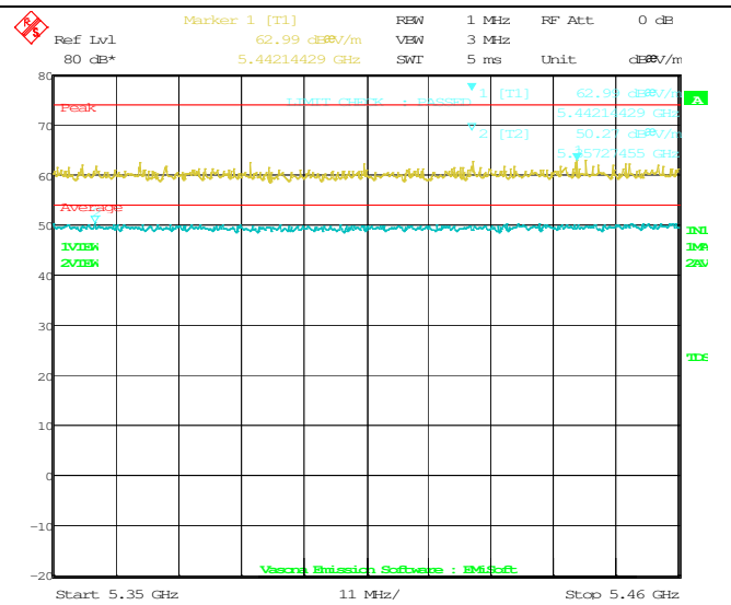
802.11n-HT20 5500M(5350-5460MHz)
