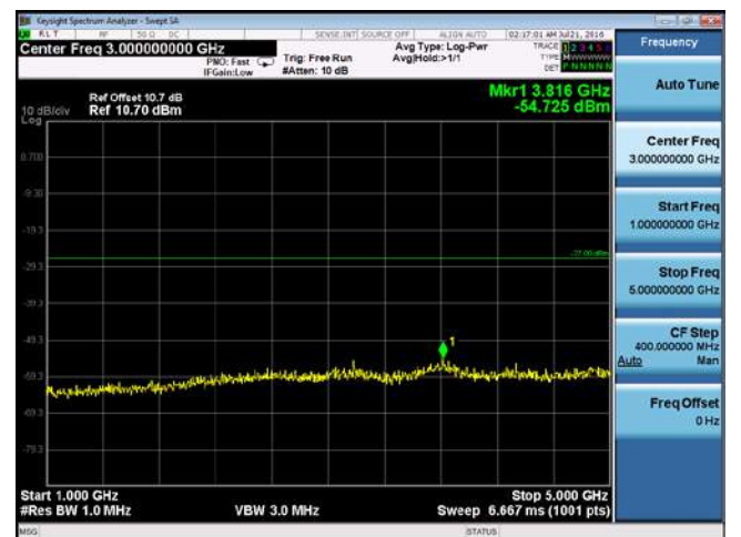
CUE-802.11n40-5710M -chain4(1GHz-5GHz)
