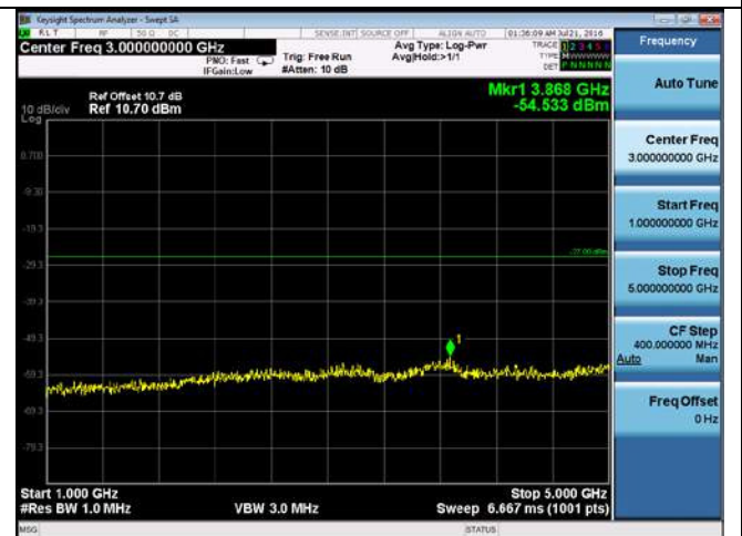
CUE-802.11ac-80-5530M -chain3(1GHz-5GHz)
