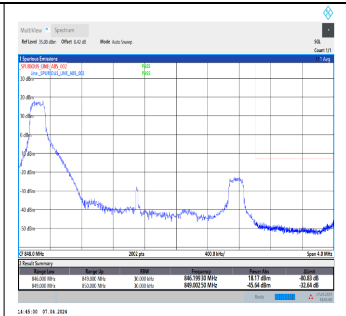
Band5_3MHz_QPSK_20635_1RB#0
