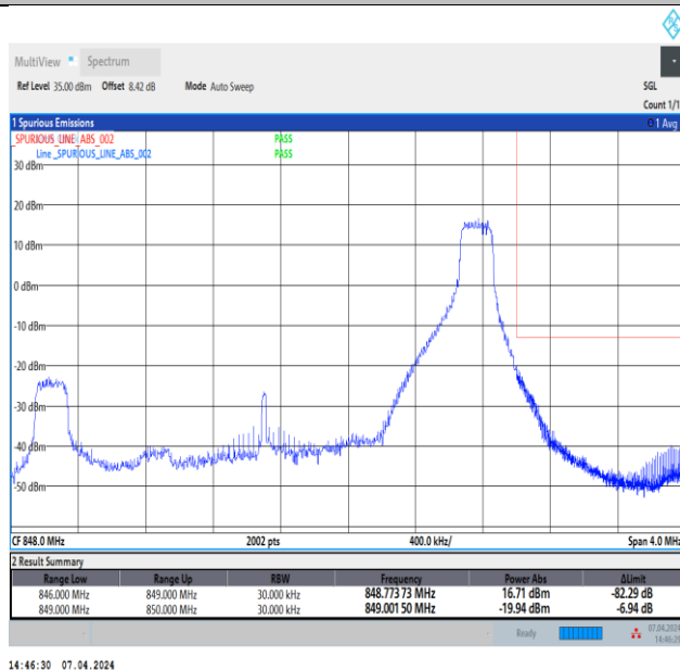
Band5_3MHz_64QAM_20635_1RB#14
