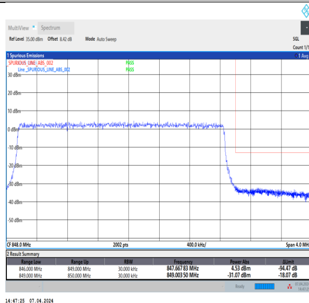
Band5_3MHz_64QAM_20635_15RB#0
