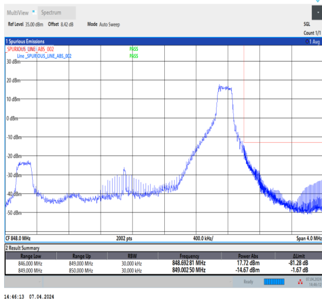
Band5_3MHz_16QAM_20635_1RB#14
