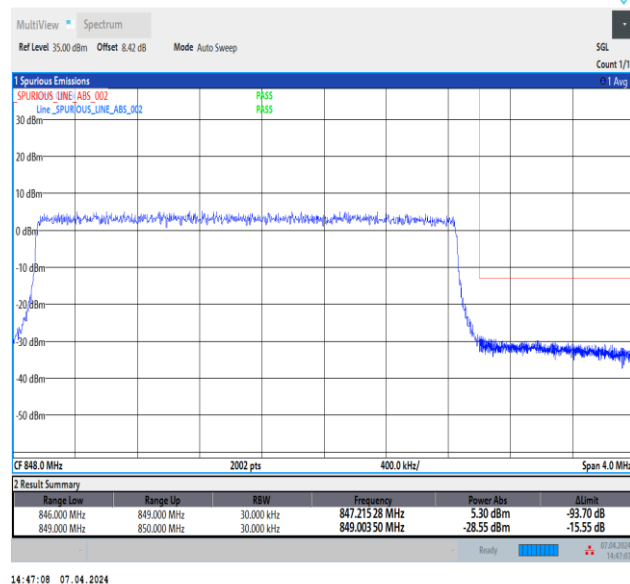
Band5_3MHz_16QAM_20635_15RB#0
