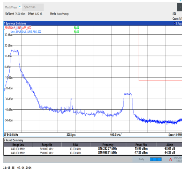
Band5_3MHz_64QAM_20635_1RB#0
