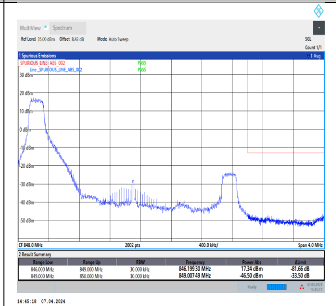
Band5_3MHz_16QAM_20635_1RB#0
