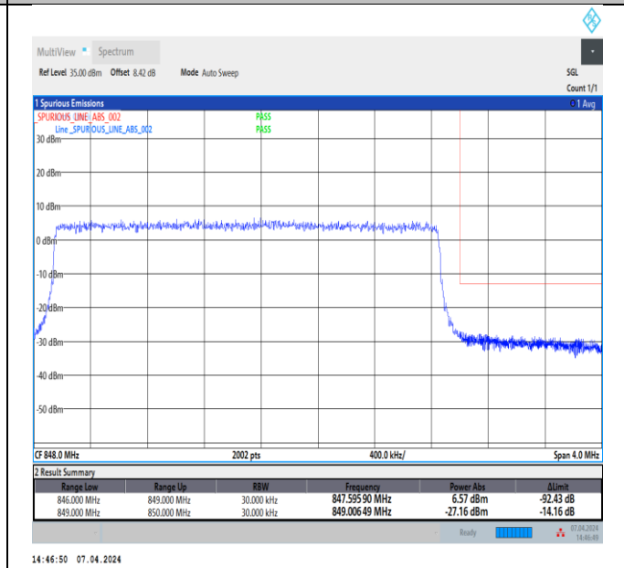
Band5_3MHz_QPSK_20635_15RB#0
