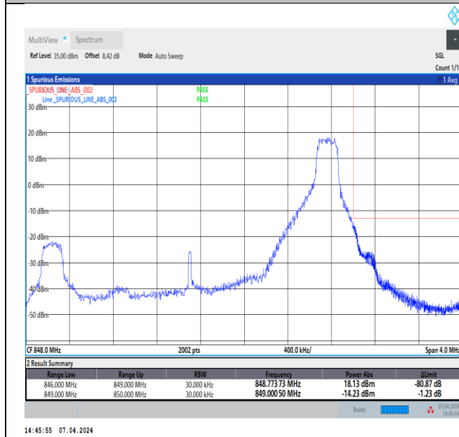
Band5_3MHz_QPSK_20635_1RB#14
