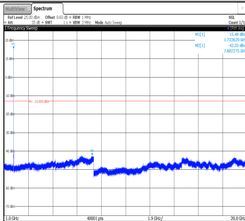
Band4-1413-5-1000~20000MHz-PASS
