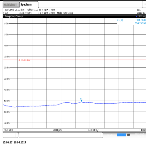
Band4-1413-4-30~1000MHz-PASS
