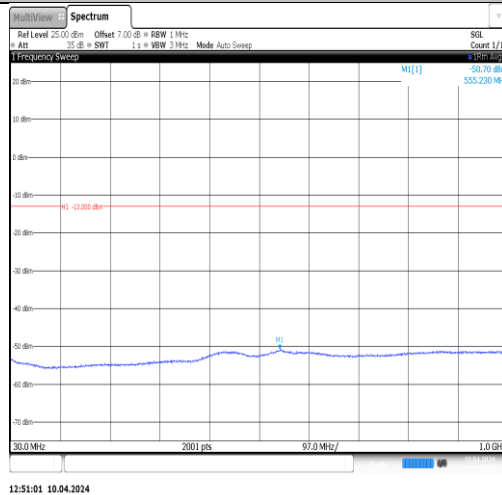
Band2-9538-5-30~1000MHz-PASS
