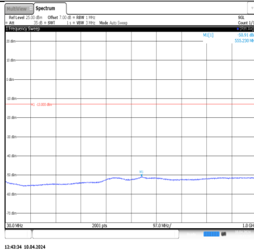
Band2-9400-3-30~1000MHz-PASS
