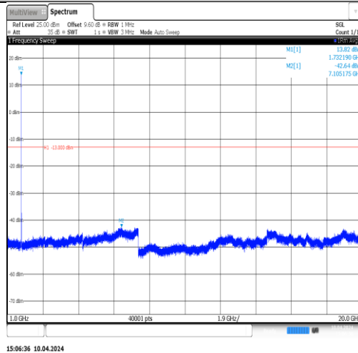
Band4-1413-4-1000~20000MHz-PASS
