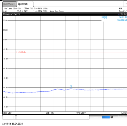
Band2-9538-3-30~1000MHz-PASS
