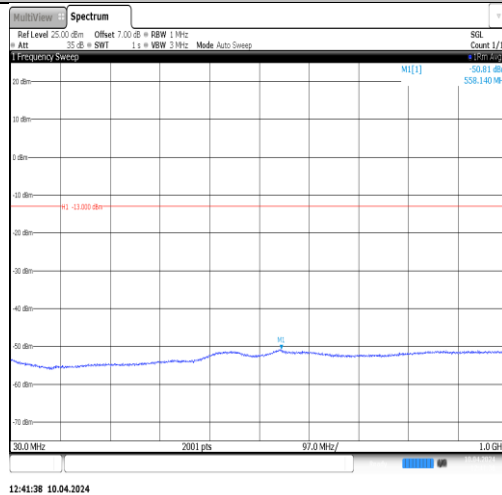
Band2-9538-2-30~1000MHz-PASS
