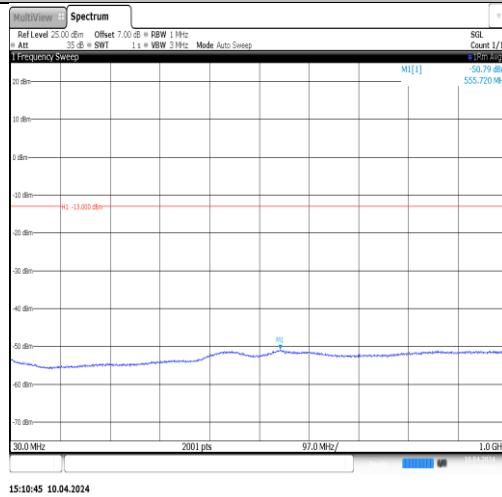
Band4-1513-5-30~1000MHz-PASS
