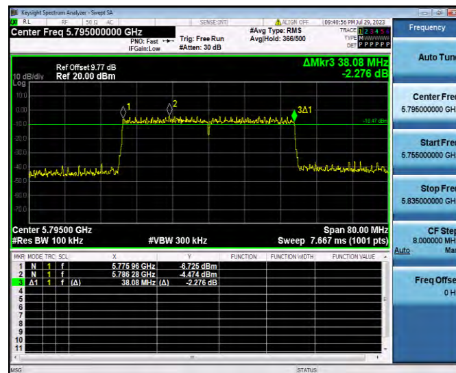
11AX40SISO_Ant0_5795
