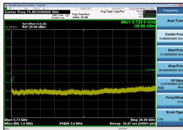
U-NII-2c ,Plot 3,5725MHz~26000MHz-802 .11ac(40MHz),5510MHz,Ant1
