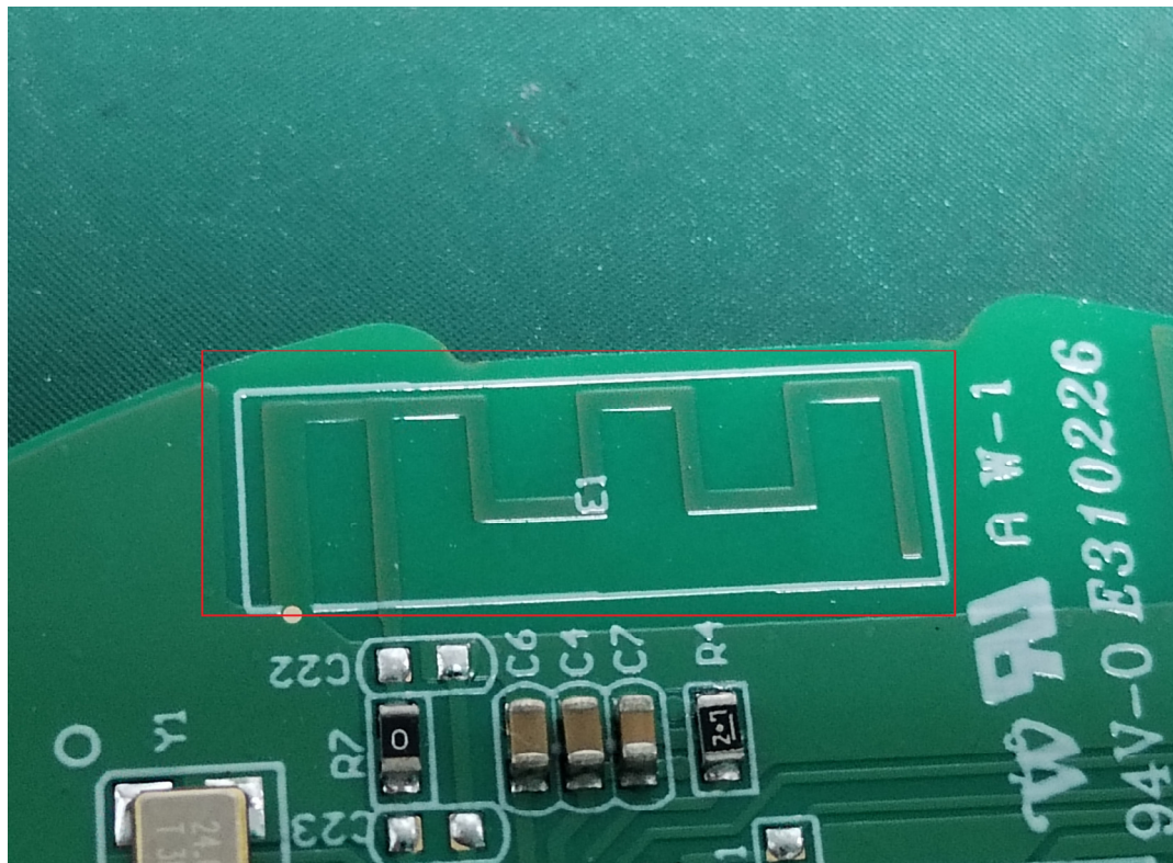
Antenna
