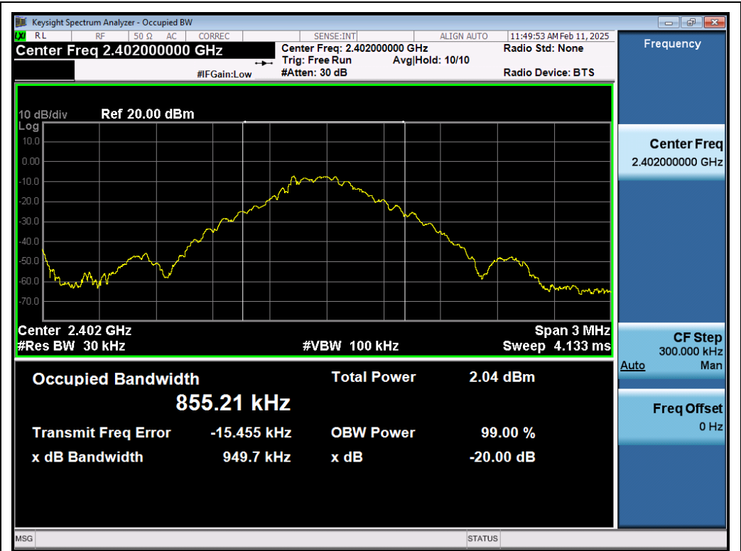
Test_Graph_BR_ANT1_2402_1Mbps_OBW
