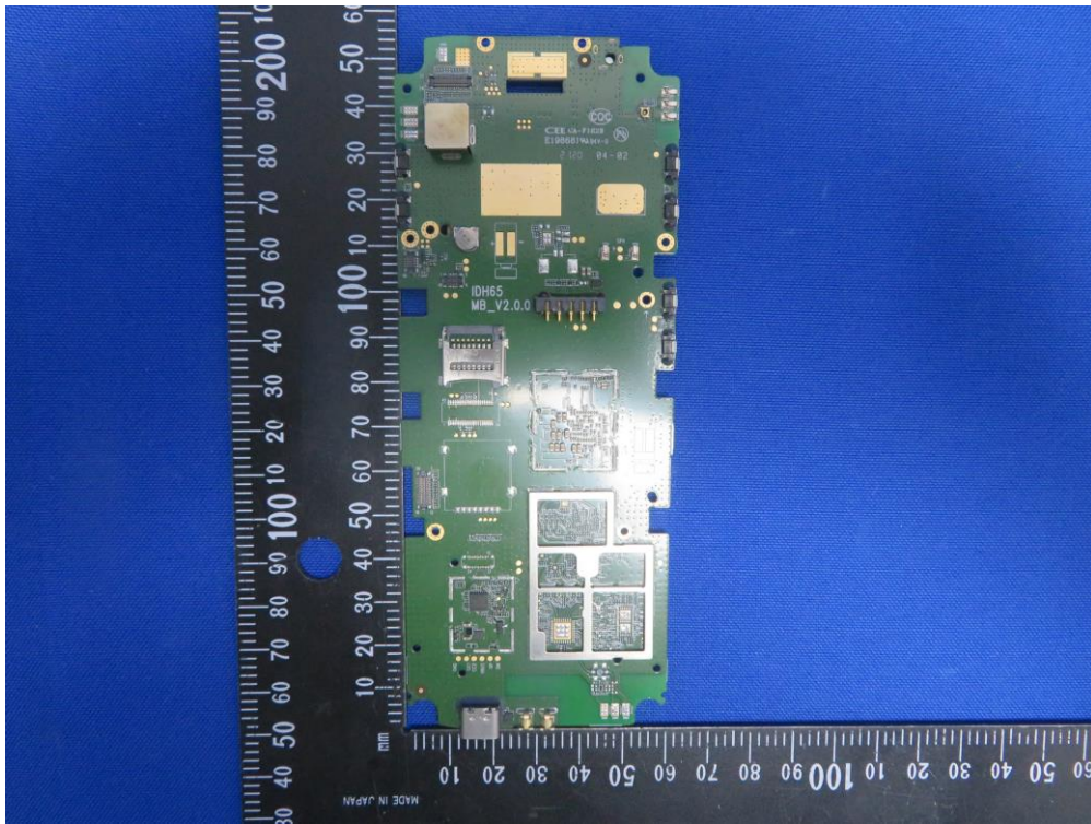
(9) EUT Photo
