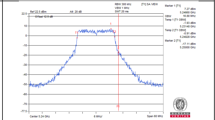
802.11a_Chain 3 / CH48
