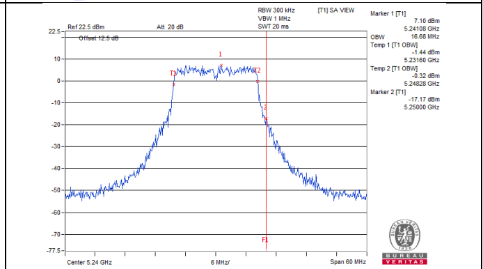
802.11a_Chain 7 / CH48
