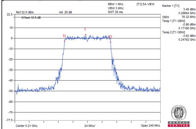
802.11ac (VHT80+80)_Chain 4 / CH42
