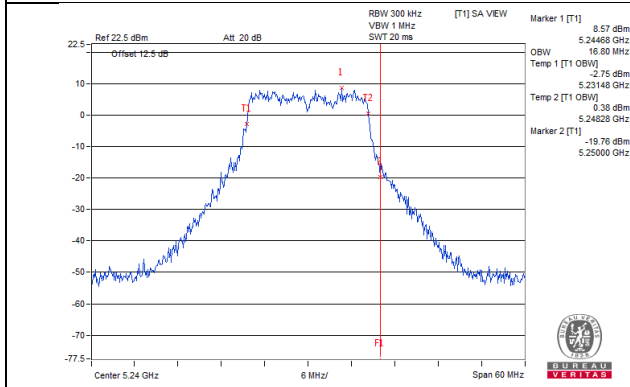
802.11a_Chain 2 / CH48
