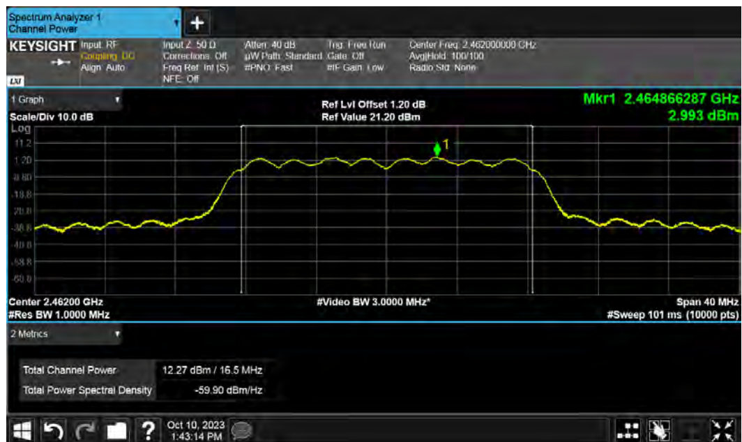
802.11g CH11
