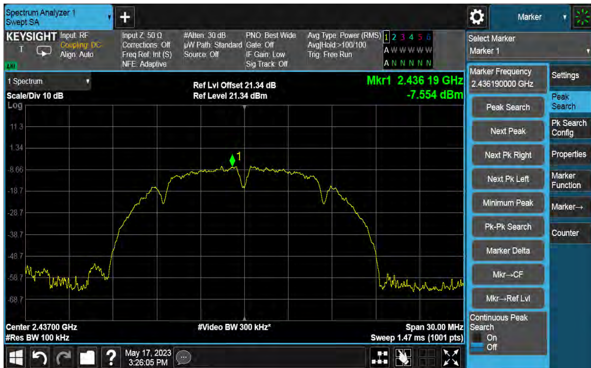
802.11b CH6
