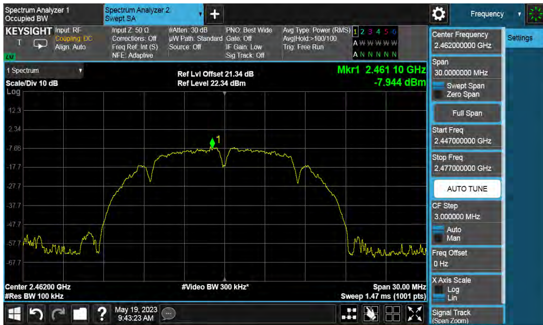
802.11b CH11
