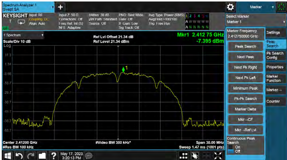
802.11b CH1
