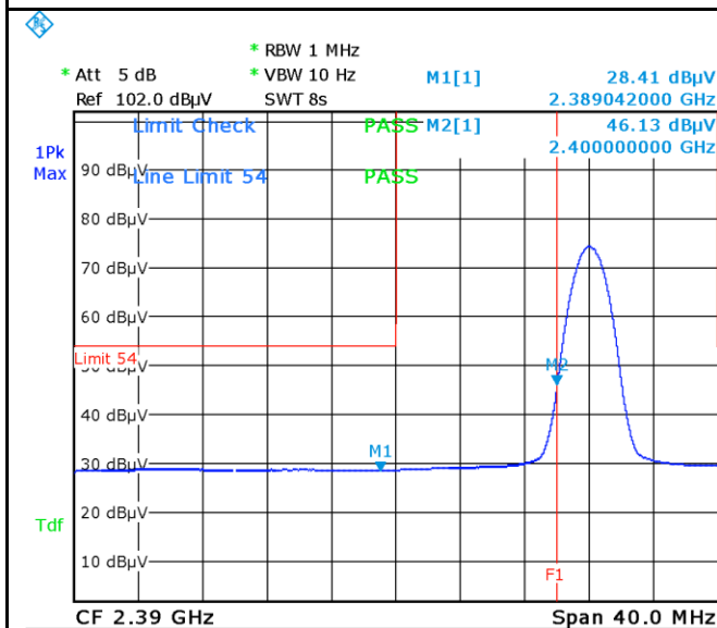
GFSK-Left Side-AV
