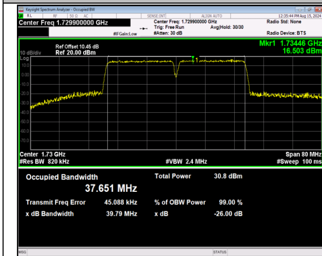
66-66-20MHz-20MHz-16QAM-16QAM-132072-132270-10 ORB#0-100RB#0-PASS
