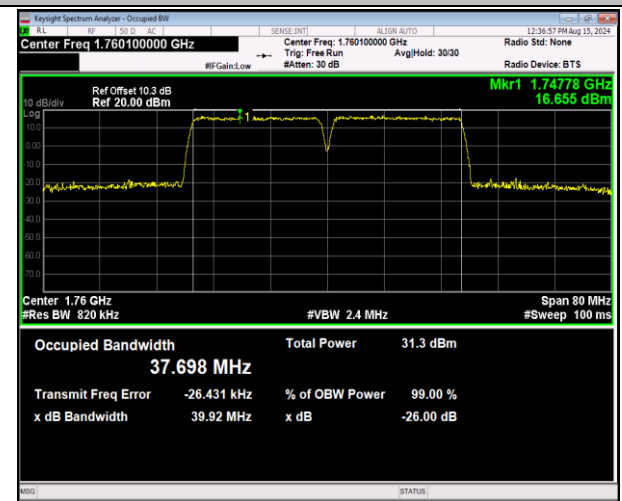
66-66-20MHz-20MHz-QPSK-QPSK-132374-132572-100R B#0-100RB#0-PASS
