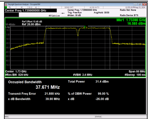
66-66-20MHz-20MHz-QPSK-QPSK-132072-132270-100R B#0-100RB#0-PASS
