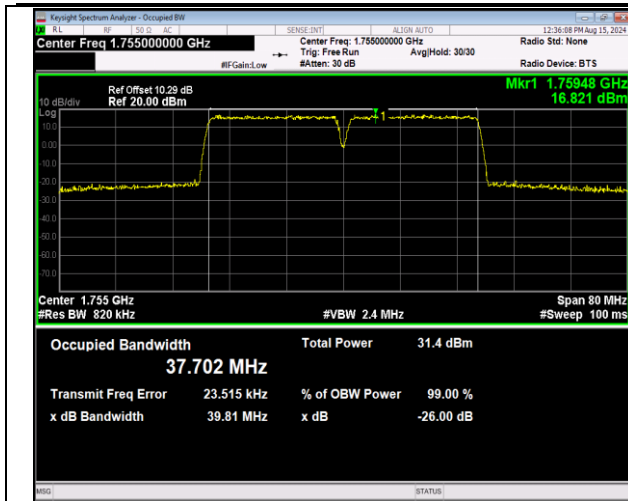
66-66-20MHz-20MHz-QPSK-QPSK-132323-132521-100R B#0-100RB#0-PASS
