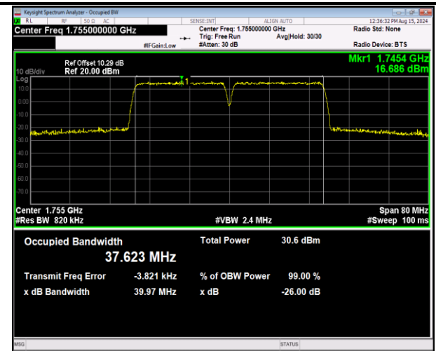
66-66-20MHz-20MHz-16QAM-16QAM-132323-132521-10 ORB#0-100RB#0-PASS
