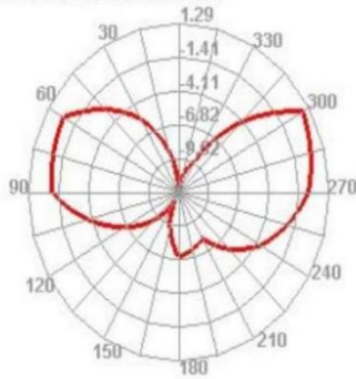
2450.000MHz H
