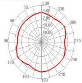
2400.000MHz H
