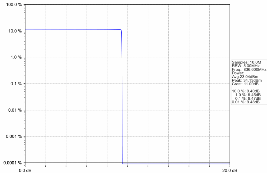
GSM850_GSM_MCH_836.6MHz_GSM_NTNV
