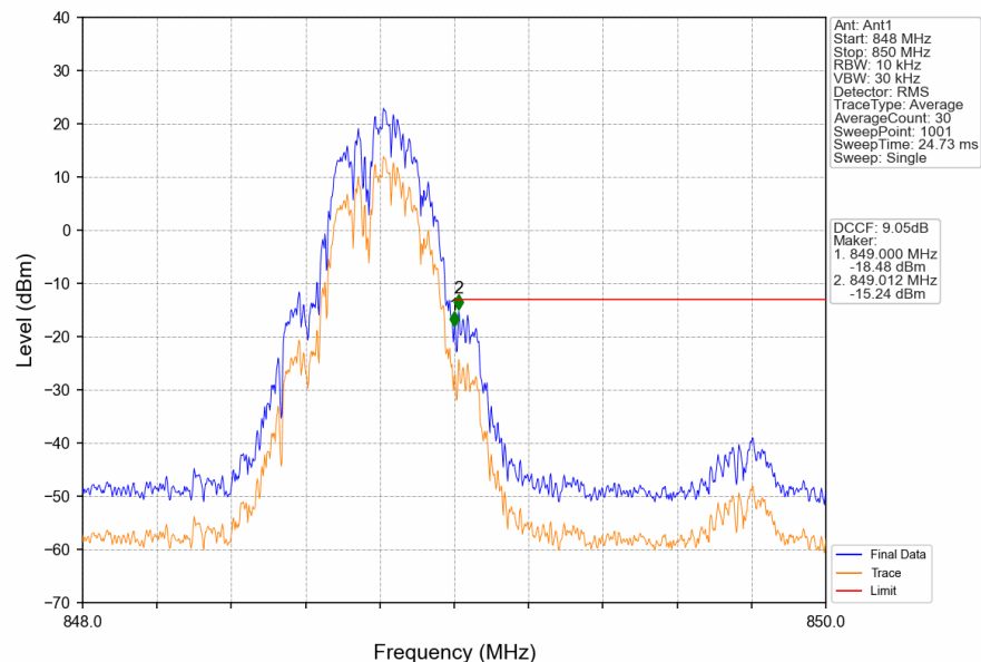
GSM850_GSM_HCH_848.8MHz_GSM_NTNV
