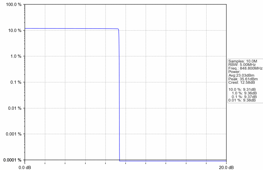
GSM850_GSM_HCH_848.8MHz_GSM_NTNV
