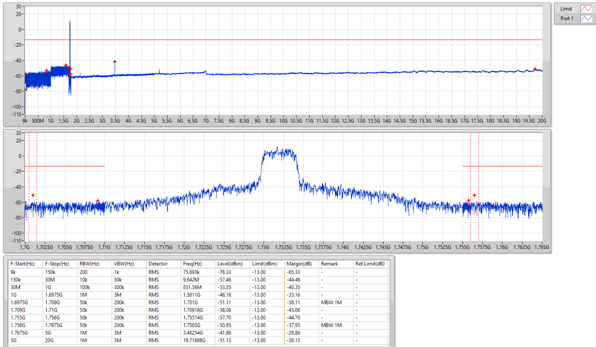
Band 4_WCDMA_5MHz_Nss1_1TX 1732MHz
