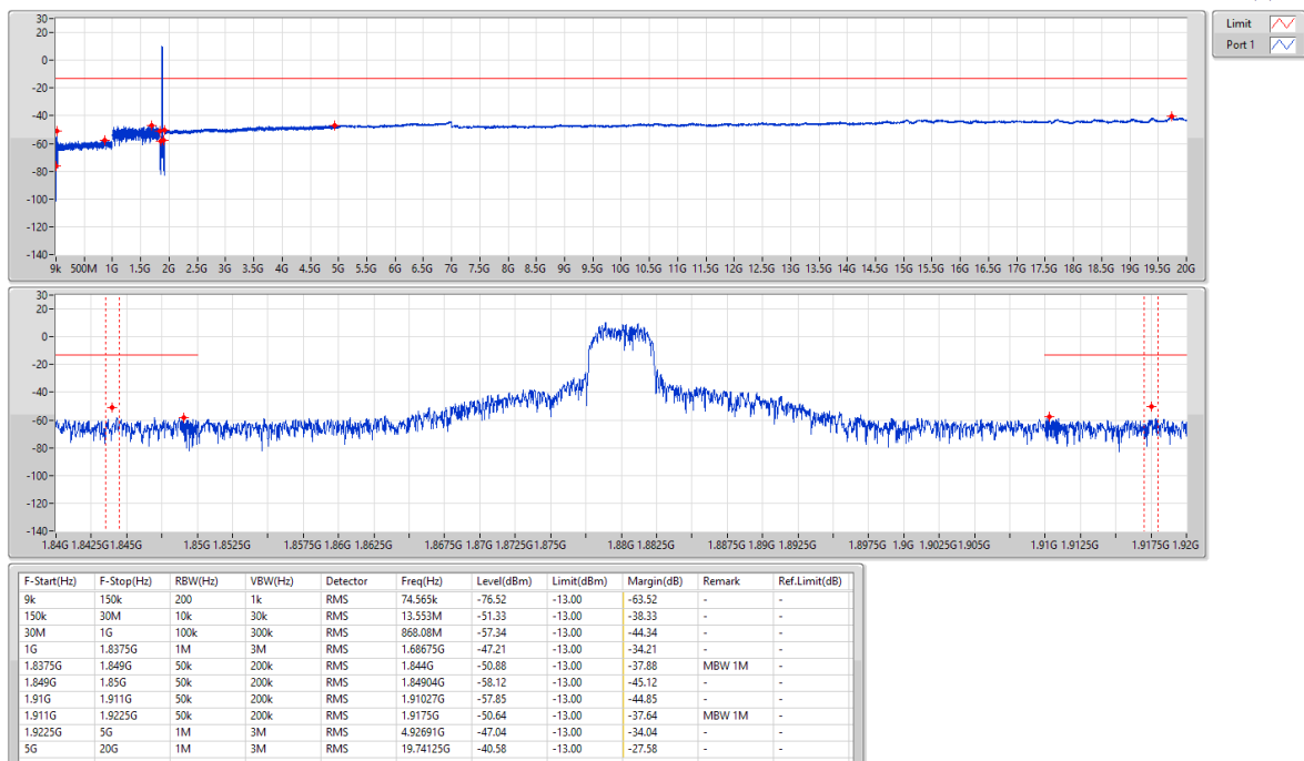
Band 2_WCDMA_5MHz_Nss1_1TX 1880MHz
