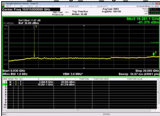
N77(15M)_DFT-s- OFDM BPSK Edge 1RB Right Low CH
