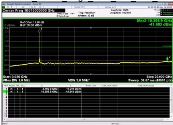
N77(90M)_DFT-s-OFDM QPSK Edge 1RB Left Low CH
