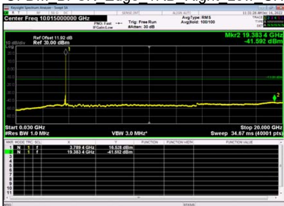
N77(90M)_DFT-s-OFDM BPSK Edge 1RB Right Low CH
