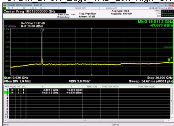
N77(100M)_DFT-s-OFDM BPSK Edge 1RB Left High CH
