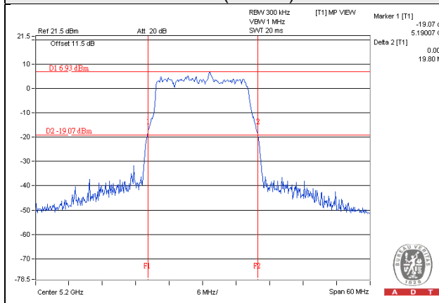
WHDI (20MHz)
