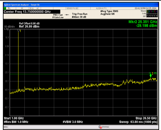
Band7-5MHz-QPSK-20775-1RB#0-Range2:1000~26500MHz
