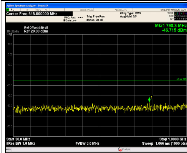
Band7-20MHz-QPSK-21100-1RB#0-Range1:30~100 0MHz
