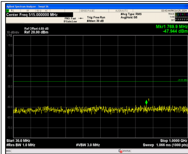
Band7-20MHz-QPSK-20850-1RB#0-Range1:30~100 0MHz
