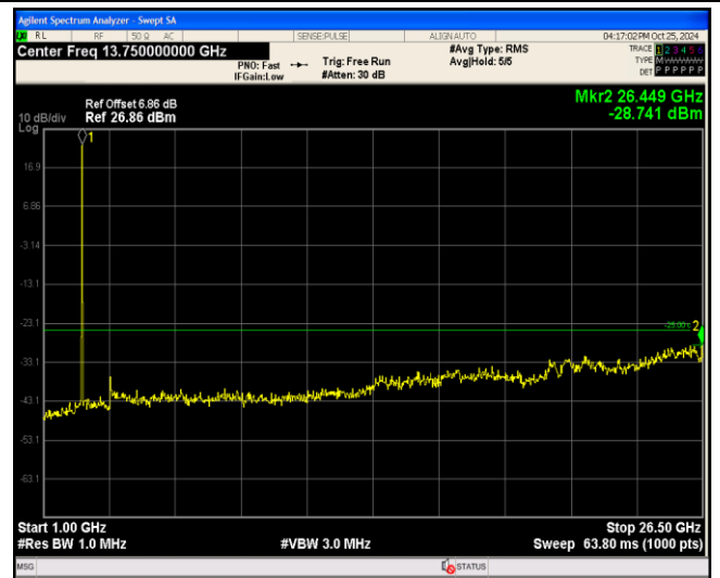
Band7-20MHz-QPSK-21100-1RB#0-Range2:1000~2 6500MHz
