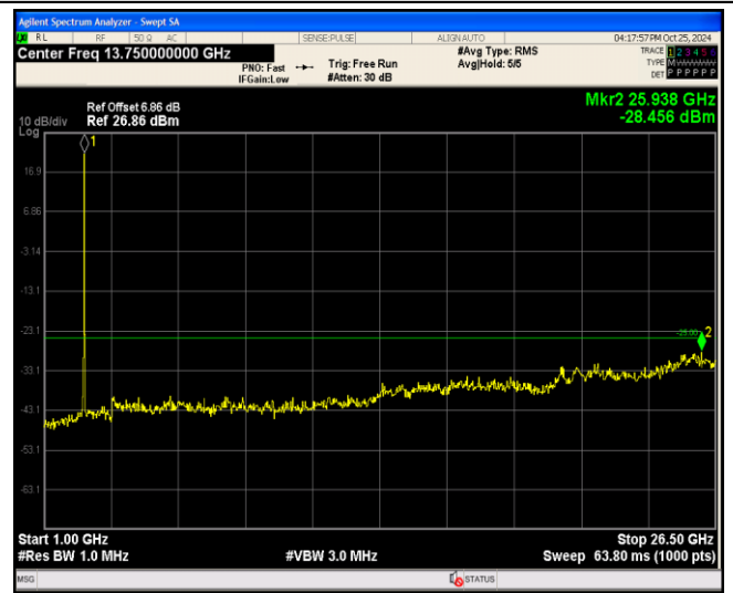
Band7-20MHz-QPSK-21100-1RB#0-Range2:1000~2 6500MHz
