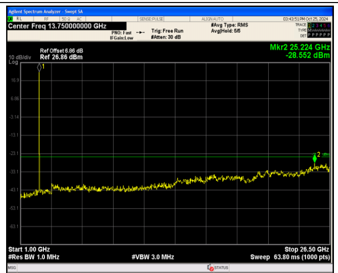
Band7-20MHz-QPSK-20850-1RB#0-Range2:1000~2 6500MHz
