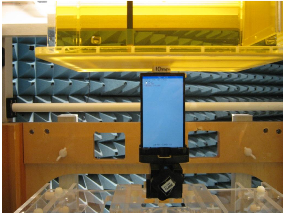
SAR - Top Edge (Body) WLAN
