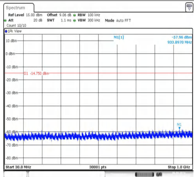
BLE_2M-Ant1-2440-30~1000-PASS
