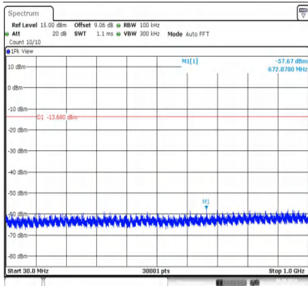
BLE_2M-Ant1-2480-30~1000-PASS
