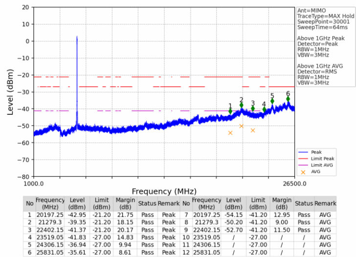
802.11ac(VHT40) HCH 5230MHz Ant 1 NTN
