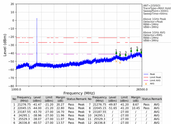
802.11a LCH 5180MHz Ant2 NTVN
