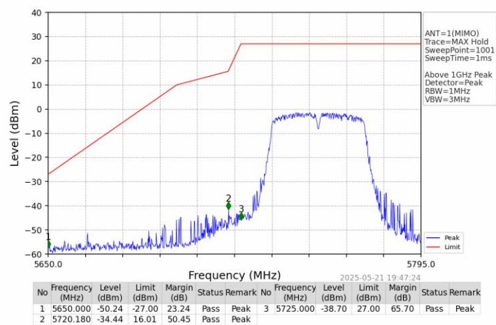
802.11ac(VHT40) LCH 5755MHz Ant1 NTN
