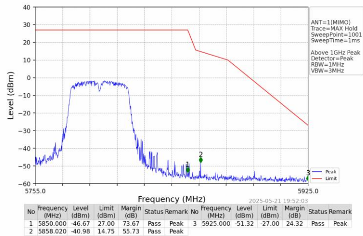
802.11ac(VHT40) HCH_5795MHz_Ant1_NTNV
