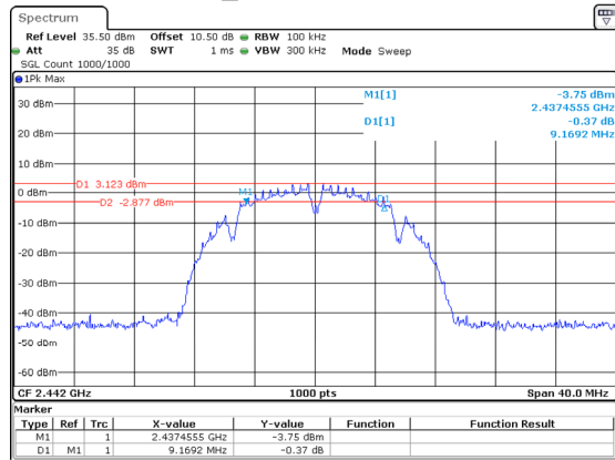
802.11b_2442MHz 9.169MHz
