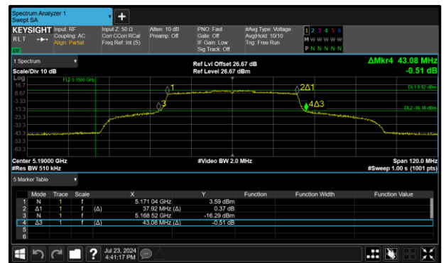
Figure 275 - 802.11ax HE40 SU Maximum 99% OBW
