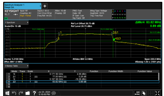
Figure 305 - 802.11ax HE80 SU Maximum 99% OBW
