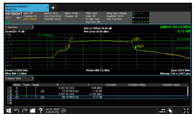
Figure 277 - 802.11ax HE80 SU Maximum 99% OBW
