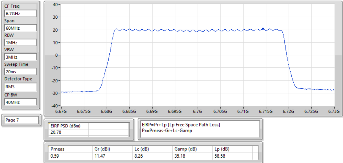
EIRP PSD;Band:6.7G;QPSK;BWch:40MHz;Nss:1;Nant:2;Ch:6700MHz;TX
