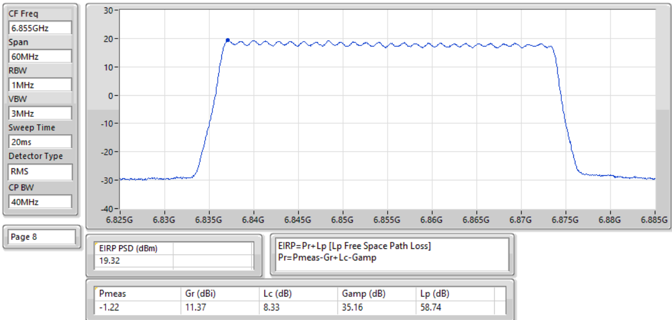
EIRP PSD;Band:6.7G;QPSK;BWch:40MHz;Nss:1;Nant:2;Ch:6855MHz;TX
