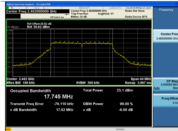
802.11n_HT20-CH 11
