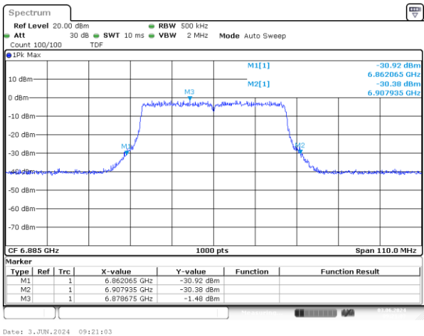
SISO-B 802.11ax/be40 ch187 26dB
