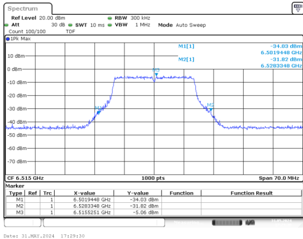
SISO-B 802.11ax/be20 ch113 26dB
