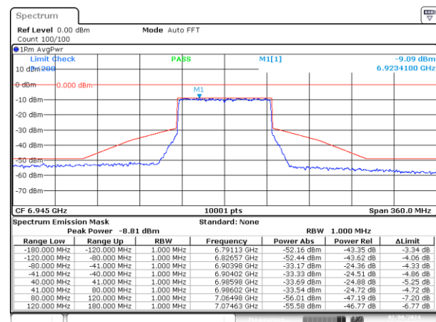
MIMO B-802.11ax/be-80MHz-Ch199-MCS0
