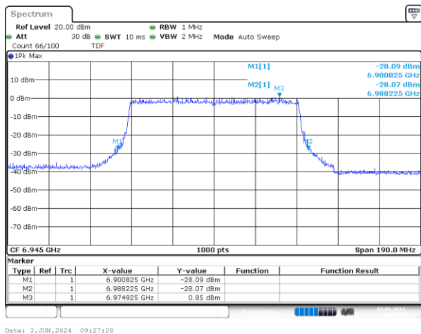
SISO-B 802.11ax/be80 CH199 26dB
