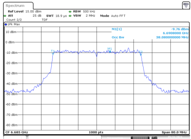
MIMO-A 802.11ax/be40 ch147 99%
