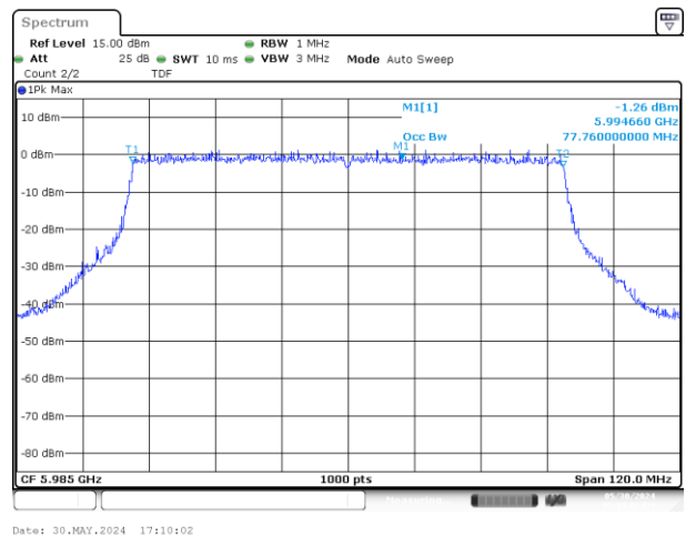
SISO-A 802.11ax/be80 ch7 99%
