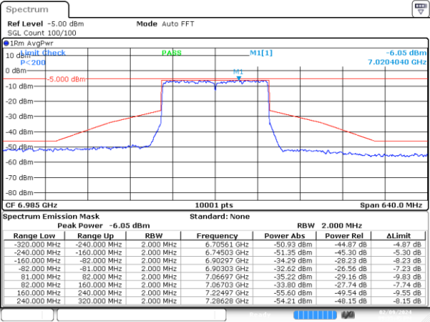
MIMO B-802.11ax/be-160MHz-Ch207-MCS0
