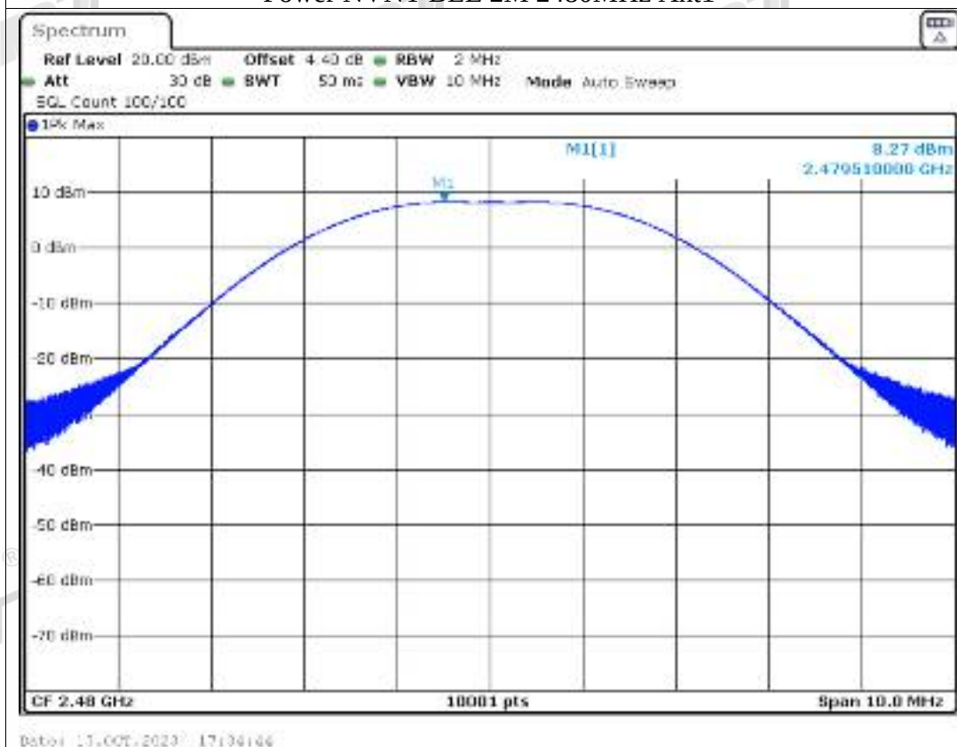
Power NVNT BLE 2M 2480MHz Ant1
