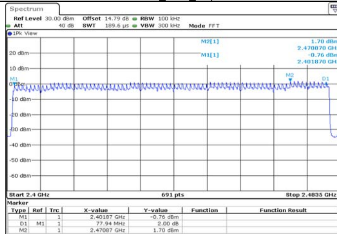
3DH1_Ant1_Hop
