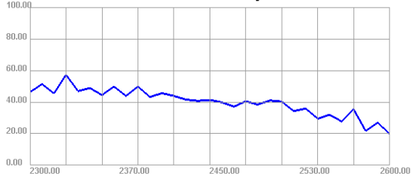
2300.00MHz - 2600.00MHz Efficiency
