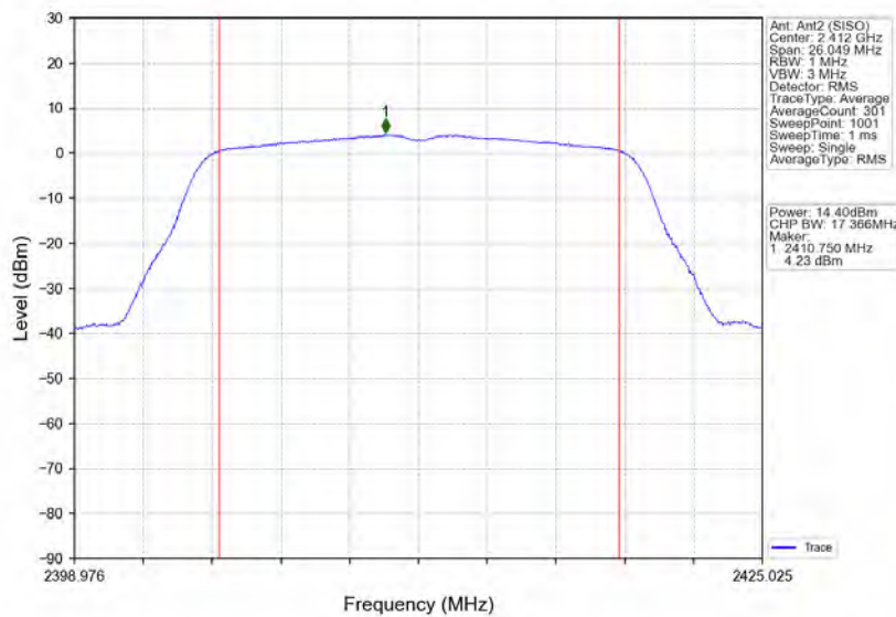
802.11g_LCH_2412MHz_Ant2 (SISO)_NTNV
