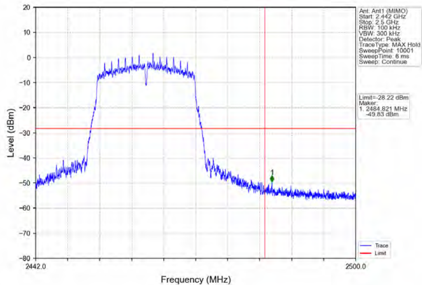
802.11n(HT20)_HCH_2462MHz_Ant1 (MIMO)_NTNV
