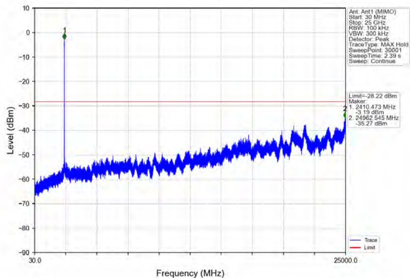
802.11n(HT20)_LCH_2412MHz_Ant1 (MIMO)_NTNV
