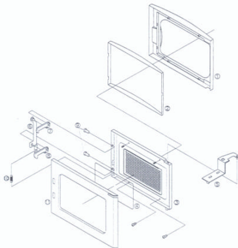
Fig. 14.3 DOOR ASSEMBLY
