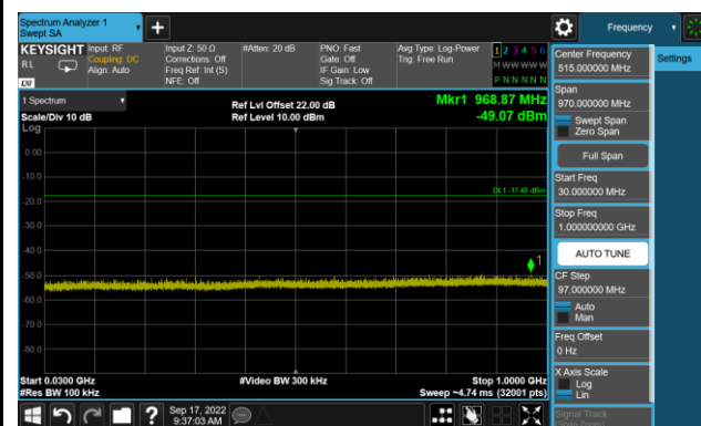
802.11 g CH01 (2412MHz)
