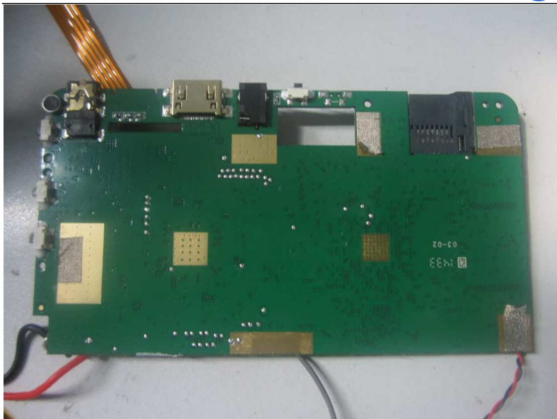
4. BT/WIFI chip view
