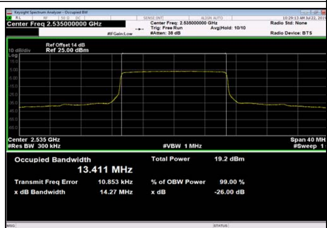
FDD07_MidRange_20_2535_Q16
