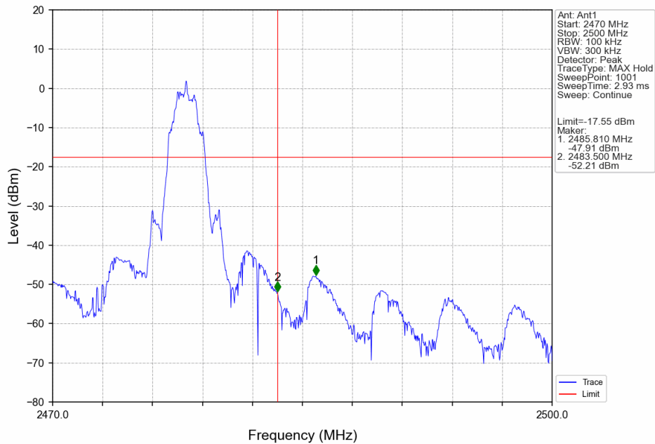
1_HCH_2478MHz_Ant1_NTNV
