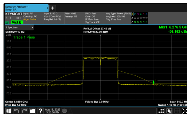
Figure 186 - A (Core 0) 802.11ax HE160 SU LPI 6025 MHz (CH15)
