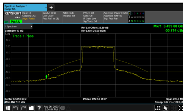
Figure 213 - A (Core 0) 802.11ax HE40 SU SP 6565 MHz (CH123)
