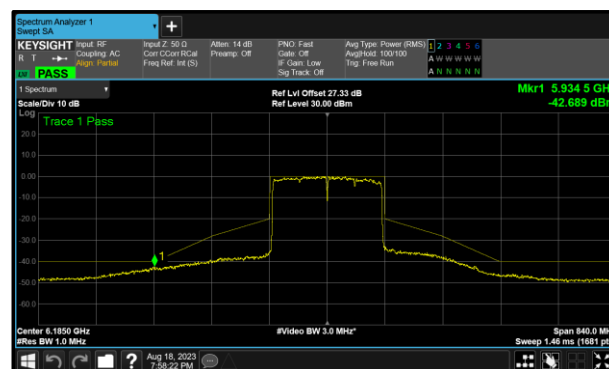
Figure 192 - B (Core 1) 802.11ax HE160 SU SP 6185 MHz (CH47)
