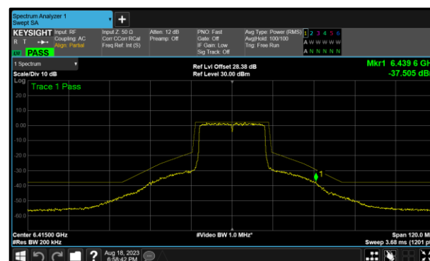
Figure 176 - A (Core 0) 802.11ax HE20 SU SP 6415 MHz (CH93)
