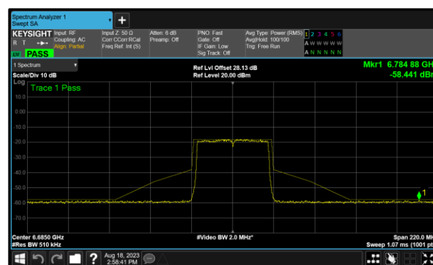
Figure 184 - A (Core 0) 802.11ax HE40 SU LPI 6685 MHz (CH147)
