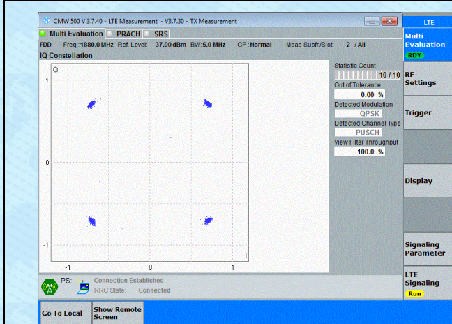
Band2-5MHz-QPSK-18900-25RB#0-PASS
