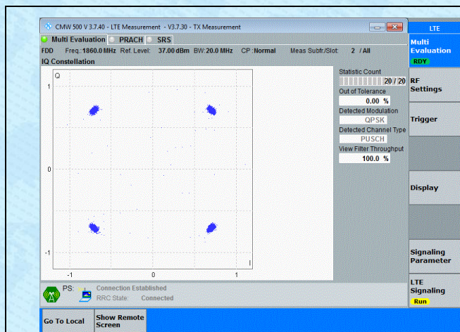
Band2-20MHz-QPSK-18700-100RB#0-PASS
