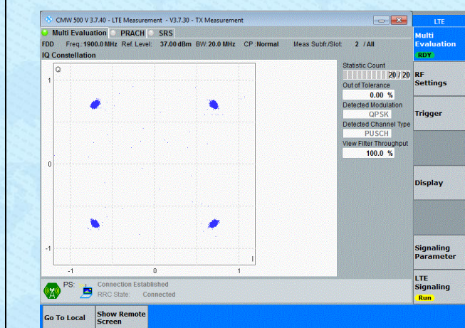
Band2-20MHz-QPSK-19100-100RB#0-PASS
