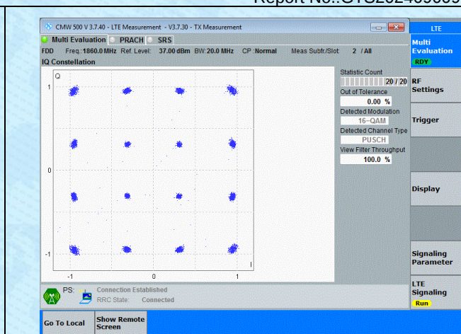
Band2-20MHz-16QAM-18700-100RB#0-PASS
