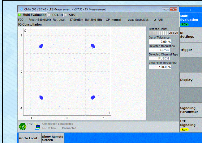
Band2-20MHz-QPSK-18900-100RB#0-PASS
