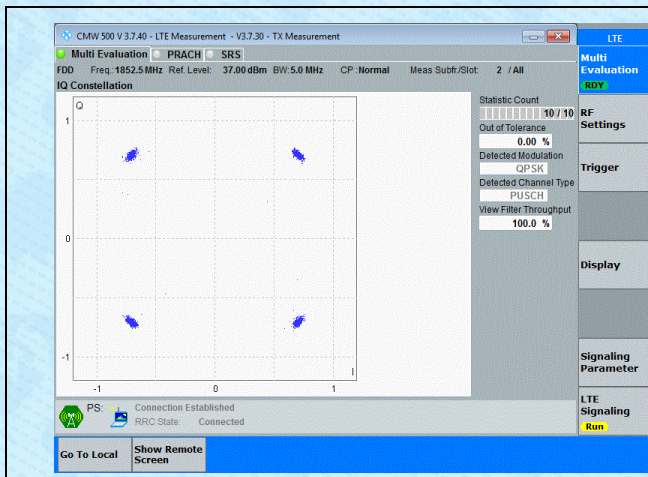
Band2-5MHz-QPSK-18625-25RB#0-PASS
