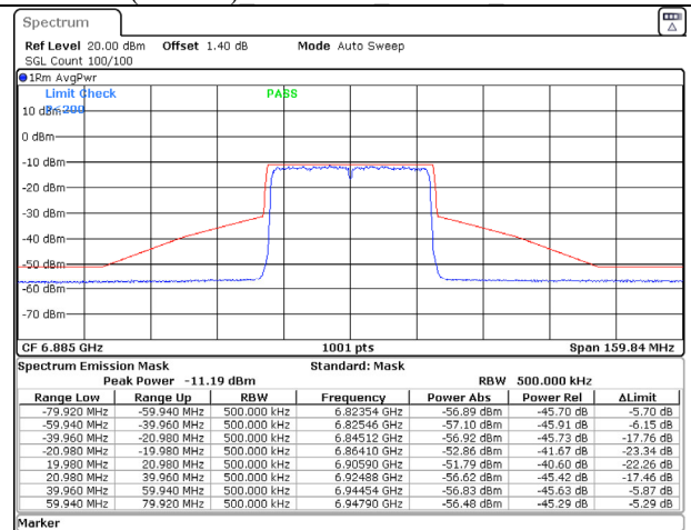
802.11ax (40MHz) 6885MHz Chain B NSS-2
