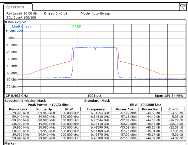
802.11ax (40MHz) 6405MHz Chain B NSS-2
