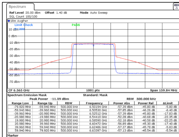
802.11ax (40MHz) 6565MHz Chain C NSS-2
