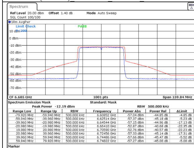
802.11ax (40MHz) 6685MHz Chain A NSS-2
