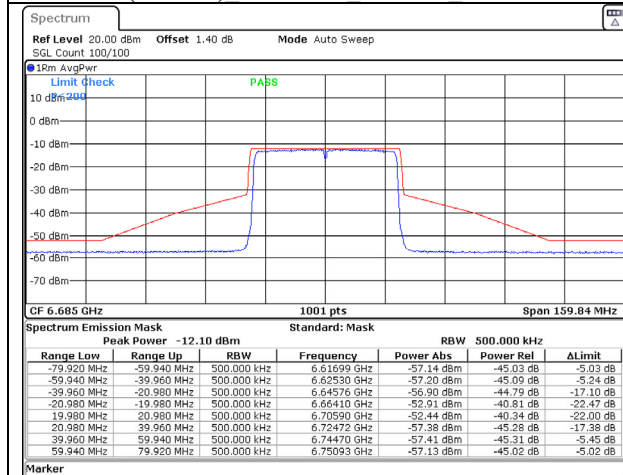
802.11ax (40MHz) 6685MHz Chain C NSS-2
