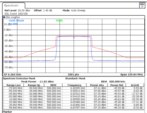
802.11ax (40MHz) 6565MHz Chain D NSS-2
