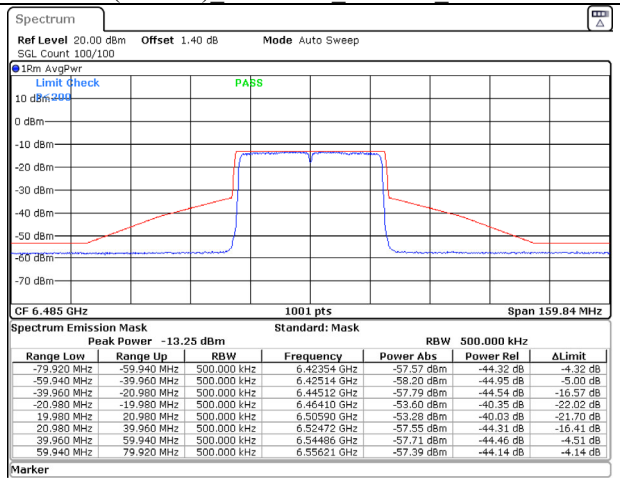
802.11ax (40MHz) 6485MHz Chain B NSS-2
