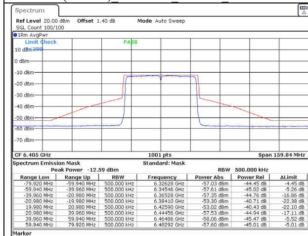
802.11ax (40MHz) 6405MHz Chain C NSS-2
