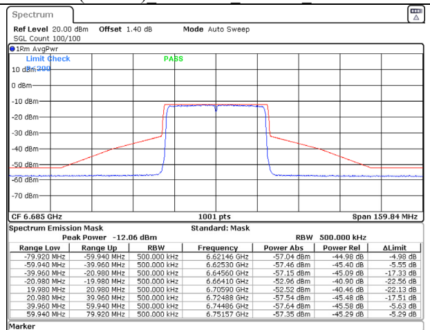
802.11ax (40MHz) 6685MHz Chain B NSS-2
