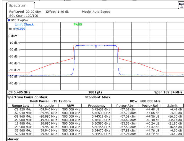
802.11ax (40MHz) 6485MHz Chain C NSS-2
