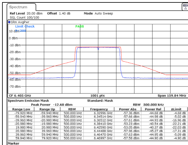
802.11ax (40MHz) 6405MHz Chain A NSS-2
