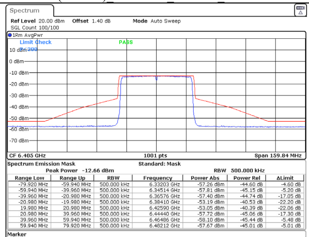
802.11ax (40MHz) 6405MHz Chain D NSS-2
