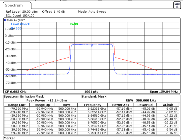
802.11ax (40MHz) 6685MHz Chain D NSS-2
