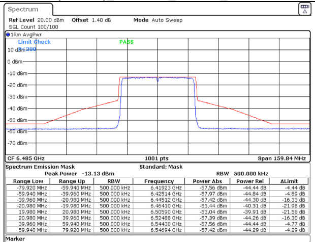
802.11ax (40MHz) 6485MHz Chain D NSS-2
