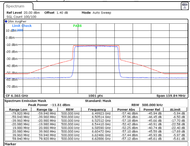
802.11ax (40MHz) 6565MHz Chain B NSS-2
